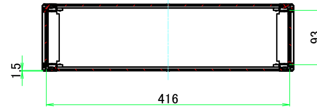
A-A ( 1 :6.5 )
