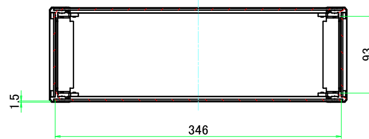
A-A ( 1 : 4.5 )
