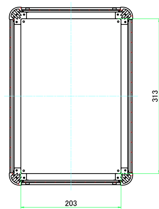
B-B ( 1 : 4.5 )
