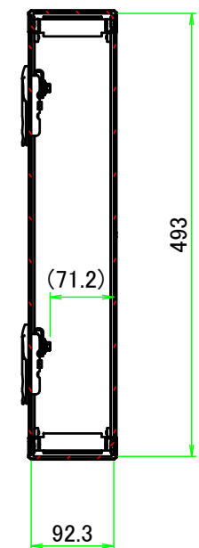
B-B ( 1 : 7.5 )
