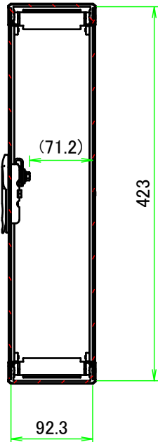
B-B ( 1 : 6 )
