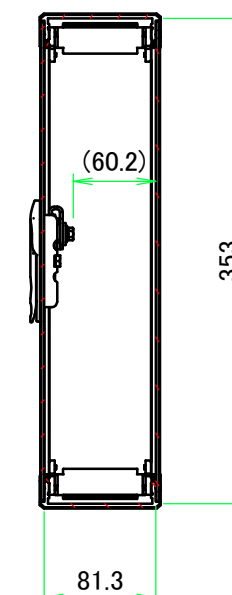
B-B ( 1 : 5.5 )
