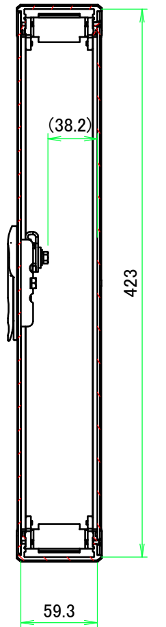
B-B ( 1 : 4 )
