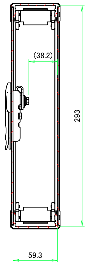
B-B ( 1 : 3 )
