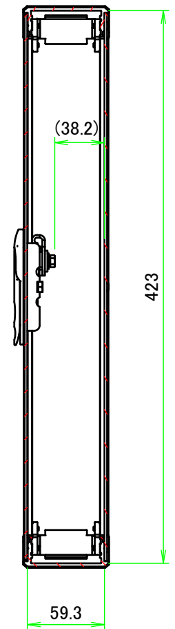
B-B ( 1 : 4 )
