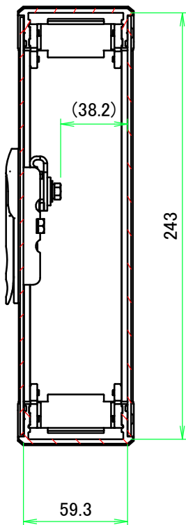
B-B ( 1 : 3 )
