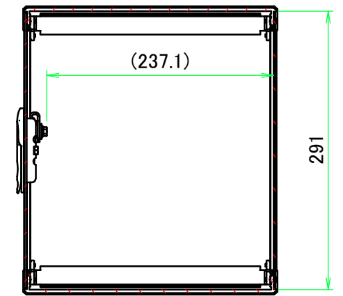
B-B ( 1 : 5.5 )
