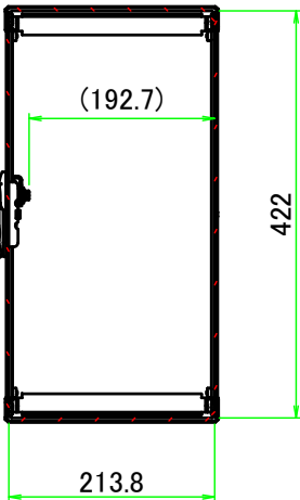
B-B ( 1 : 8.5 )
