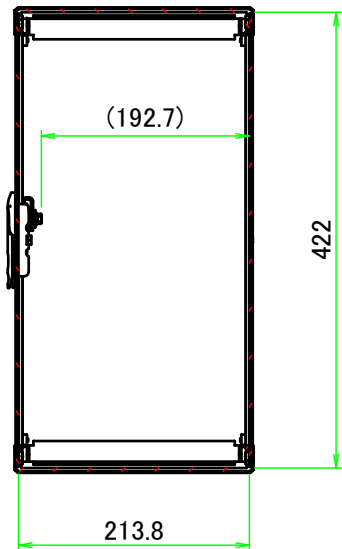
B-B ( 1 : 7 )
