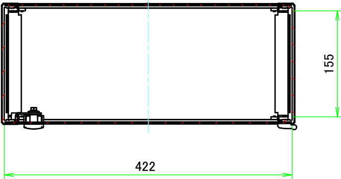
A-A ( 1 : 5.5 )
