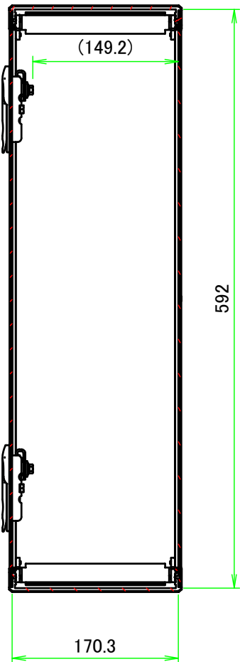
B-B ( 1 : 5.5 )
