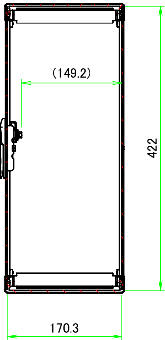
B-B ( 1 : 5.5 )
