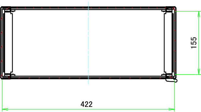
A-A ( 1 : 5.5 )
