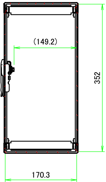
B-B ( 1 : 5.5 )
