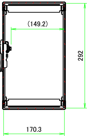
B-B ( 1 : 5.5 )
