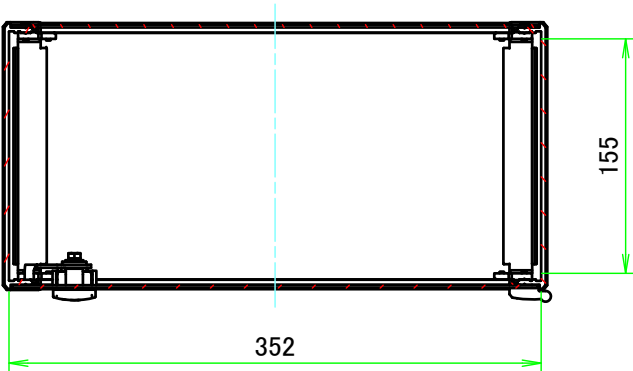
A-A ( 1 : 5 )
