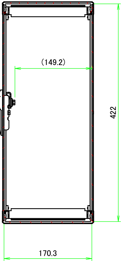
B-B ( 1 : 4.5 )
