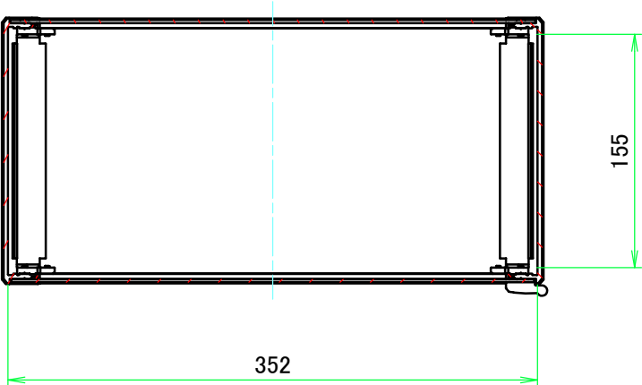
A-A ( 1 : 4.5 )
