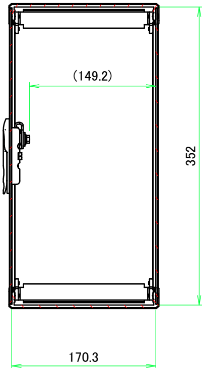
B-B ( 1 : 4.5 )
