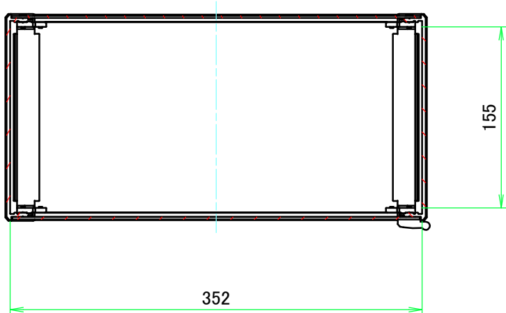
A-A ( 1 : 4.5 )
