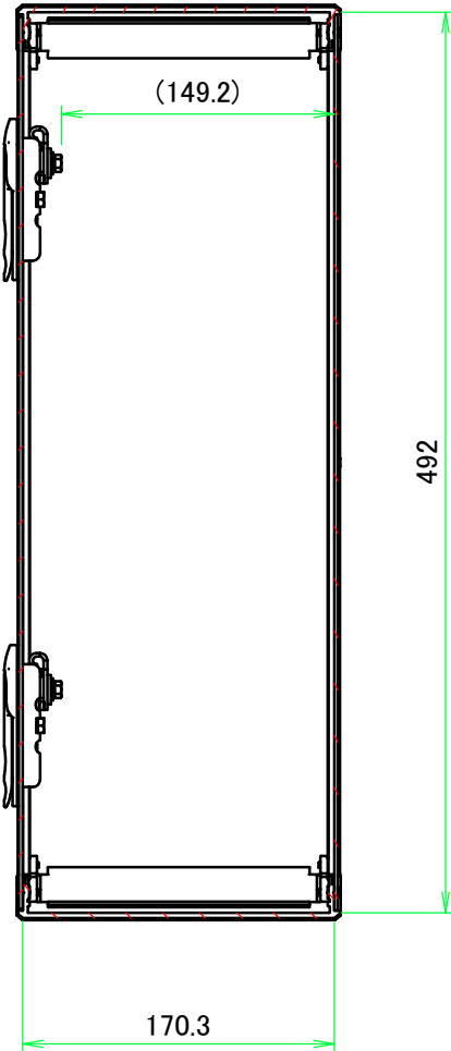
B-B ( 1 : 4.5 )
