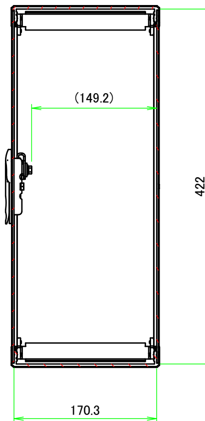
B-B ( 1 : 4.5 )
