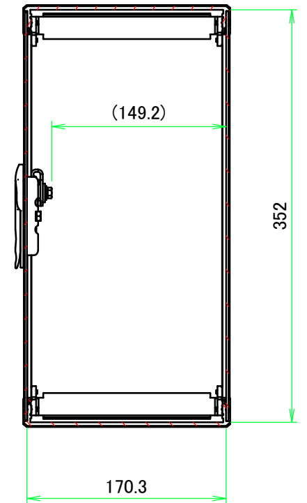
B-B ( 1 : 4.5 )
