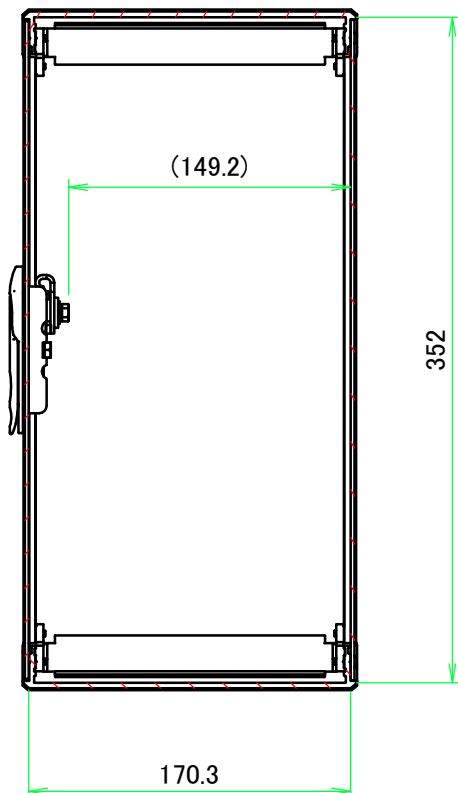
B-B ( 1 : 4 )
