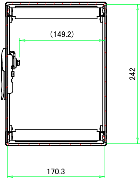
B-B ( 1 : 4 )
