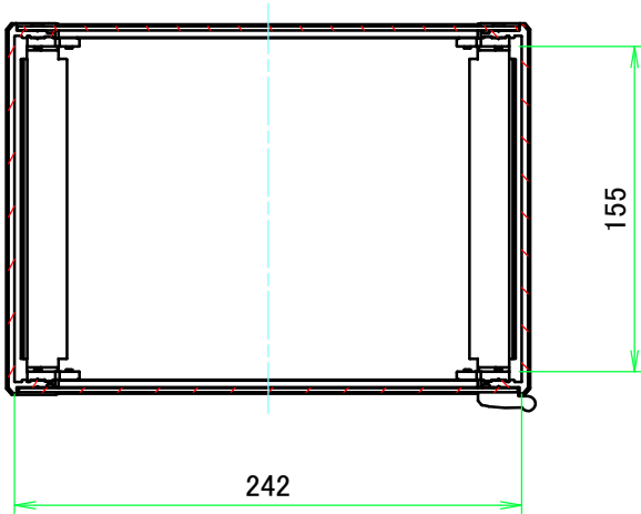
A-A ( 1 : 4 )
