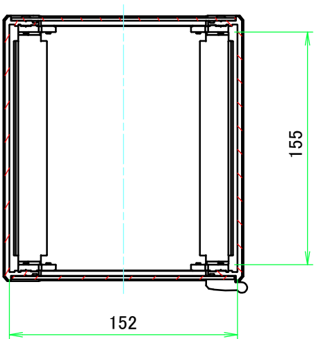
A-A ( 1 : 3.5 )
