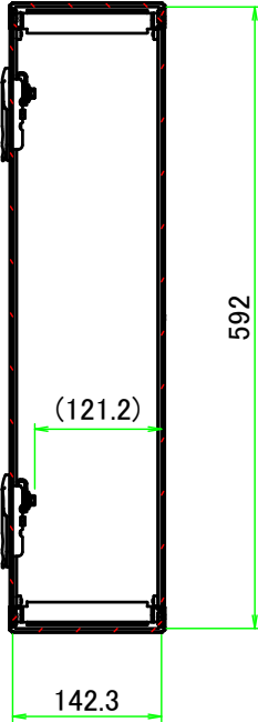
B-B ( 1 : 8 )
