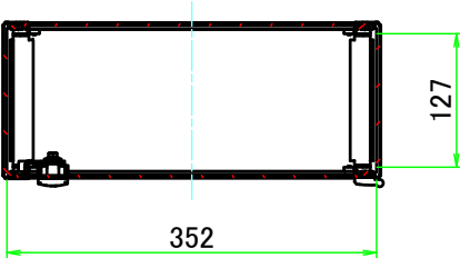
A-A ( 1 : 8 )
