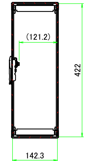
B-B ( 1 : 7.5 )
