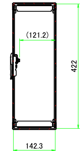
B-B ( 1 : 7.5 )
