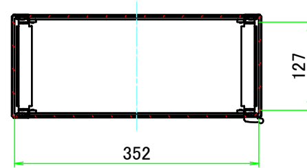
A-A ( 1 : 7.5 )
