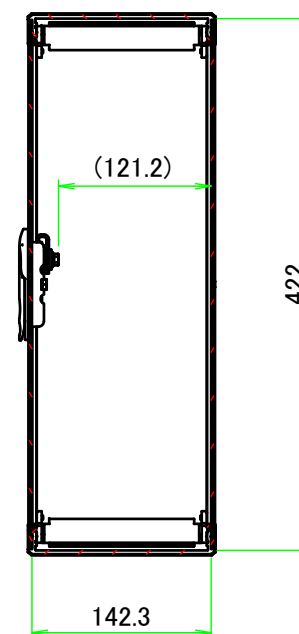
B-B ( 1 : 6 )
