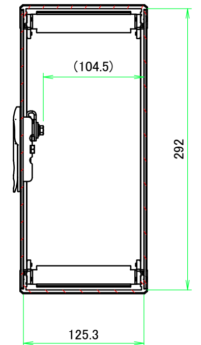
B-B ( 1 : 4 )
