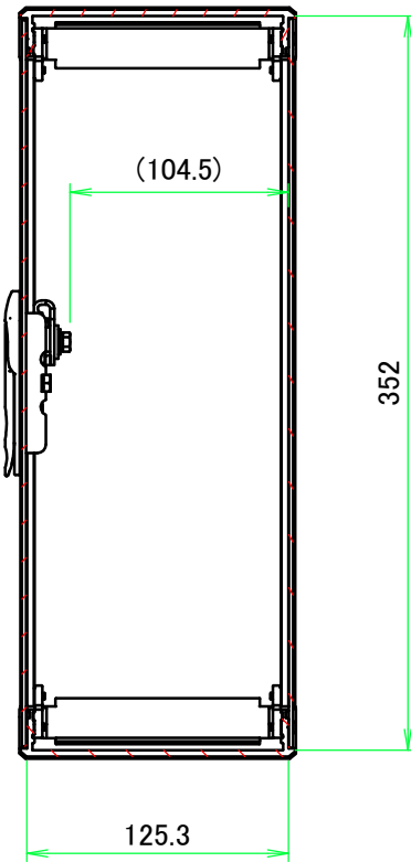
B-B ( 1 : 4 )
