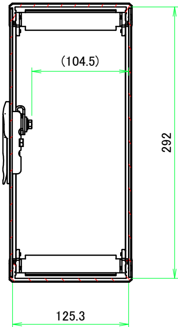
B-B ( 1 : 4 )
