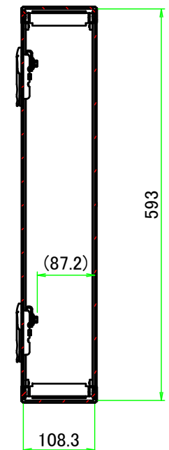
B-B ( 1 : 8 )
