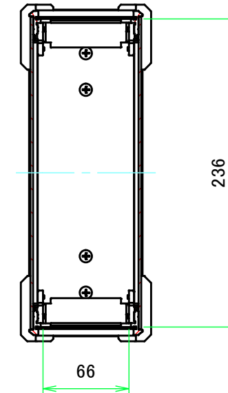
A-A ( 1:4 )
