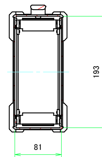
C-C ( 1:4 )
