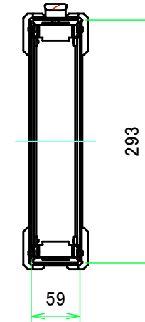
C-C ( 1:6.5 )
