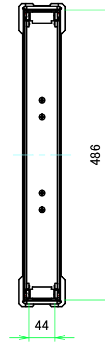
A-A ( 1:6.5 )
