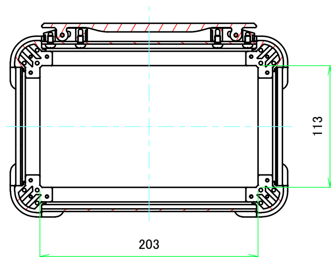
B-B ( 1:3.5 )
