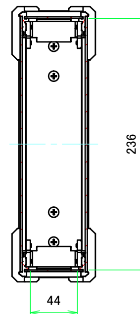
A-A ( 1:3.5 )
