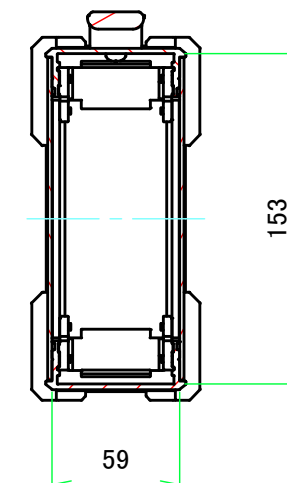
C-C ( 1:3.5 )
