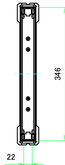
A-A ( 1:6 )
