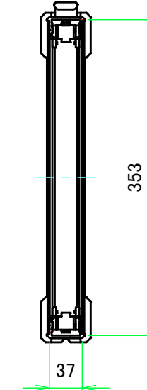
C-C ( 1:6 )
