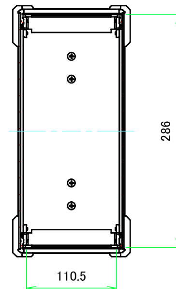
A-A ( 1:4.5 )
