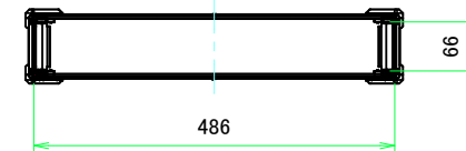
A-A (1:8)
