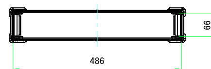
A-A (1:7.5)
