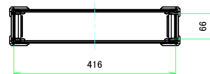
A-A (1:7)
