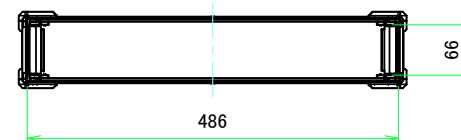
A-A (1:7)
