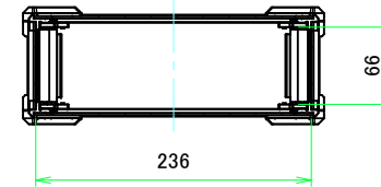
A-A (1:5)
