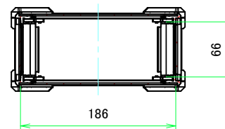
A-A (1:4.5)
