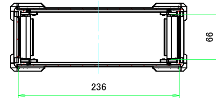
A-A (1:4)
