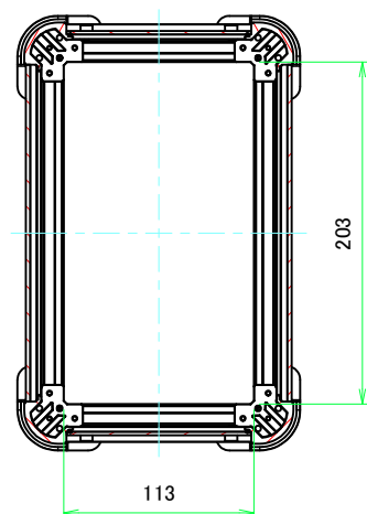
B-B (1:3.5)
