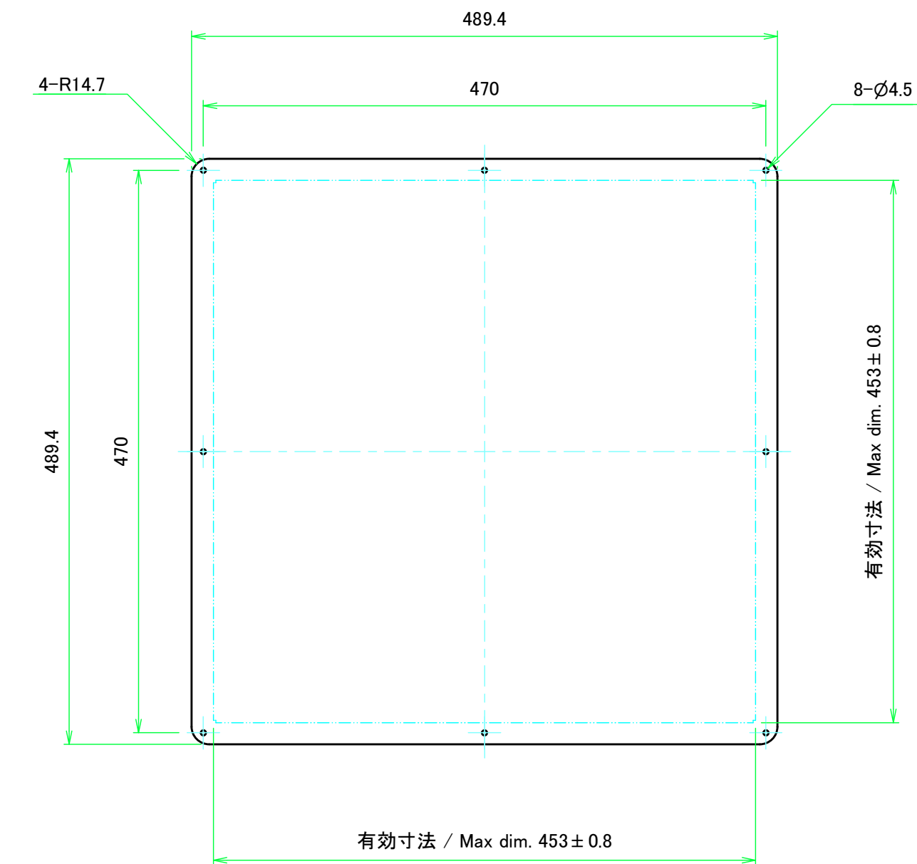
保護シート側 Surface protective film side
