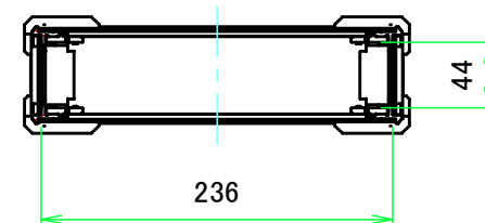
A-A ( 1:5.5 )
