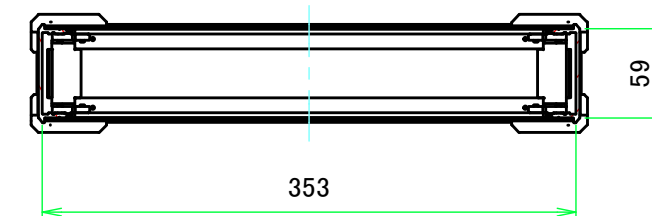
C-C ( 1:5 )
